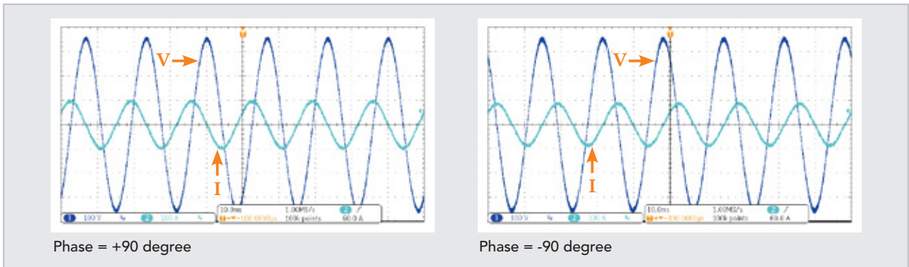
CC相位超前/落后模式
