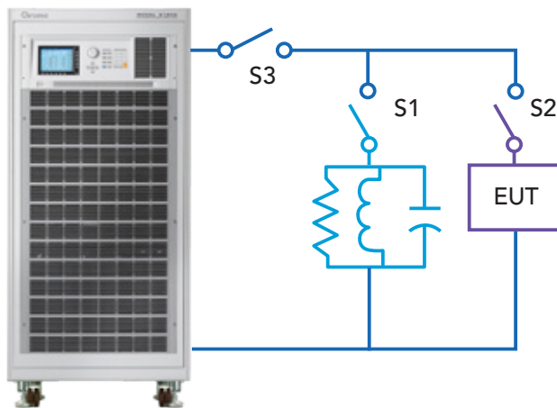
61800系列 回收式电网模拟电源
