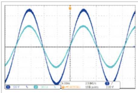
CC整流模式 (CF=1.414)
