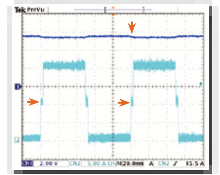
图 4：并联非同步动态负载
