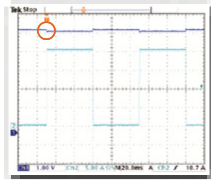
图 3：并联同步动态负载
